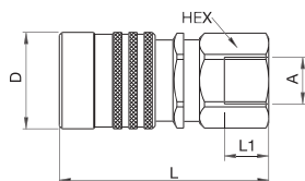
Внутренняя резьба
