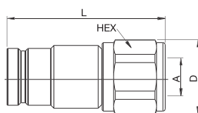
Внутр. резьба
