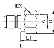
Внутр. резьба
