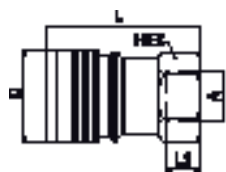
Внутр. резьба
