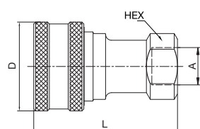
Внутр. резьба
