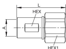
Внутр. резьба
