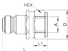
Внутренняя резьба
