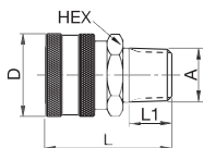
Наружн. резьба
